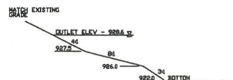
SECTION D D'
